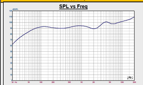
频响曲线
