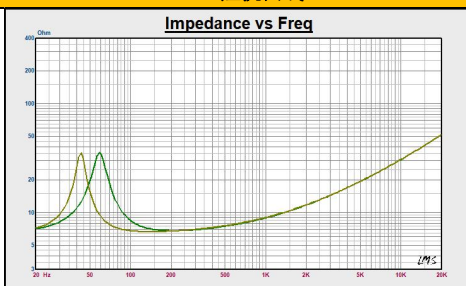
阻抗曲线
