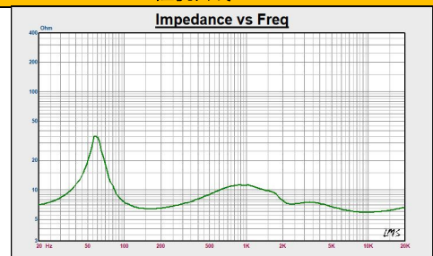
阻抗曲线
